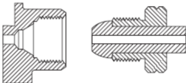
CGA 590 .965-14NGO-LH-INT
