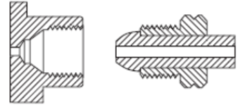
CGA 510 .885-14NGO-LH-INT (Bullet Nipple)
