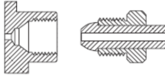
CGA 500 .885-14NGO-RH-INT (Bullet Nipple)
