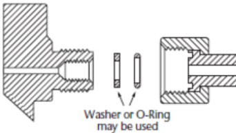
CGA 180 .625-18UNF-2A-RH-EXT
